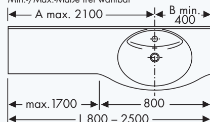
Beckenplatzierung innerhalb der Min./Max.-Maße frei wählbar
