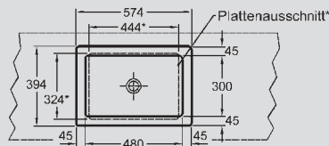
Washtop® E classic Aufsatzwaschtisch 574 x 394 mm, mit Standardablauf, Modell-Nr. 405574.
