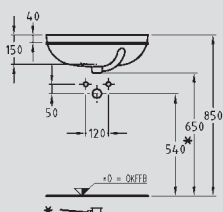
Ovin 10 Modell-Nr. 244053 mit Überlauf Modell-Nr. 244055 ohne Überlauf
