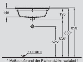
Renona Nr. 1 Plan Modell-Nr. 242150 Modell-Nr. 242155 außen glasiert
